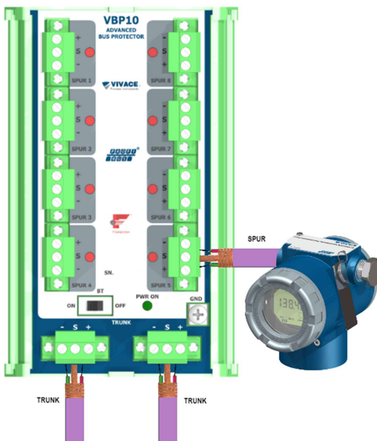
Figura 2.4 – Conexões e descrição dos terminais do VBP10.
