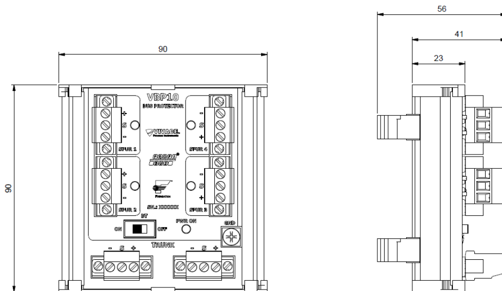
Figura 2.1 – Desenhos dimensionais do VBP10, modelo 4 canais.
