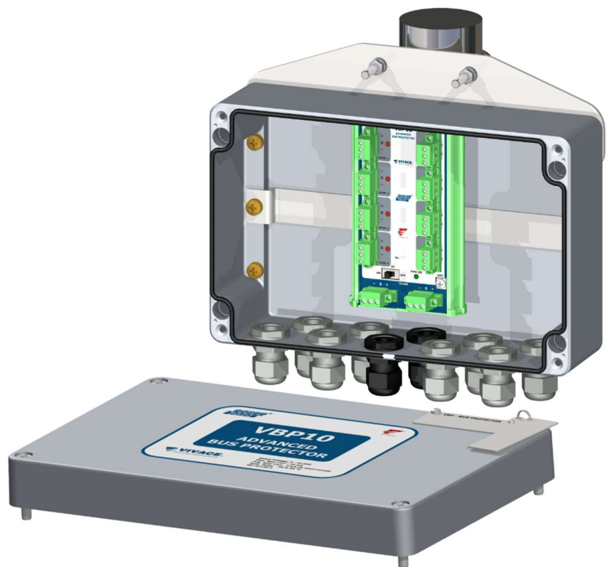
Figura 5.2 – Caixa de proteção do VBP10 (modelo 8 canais).
