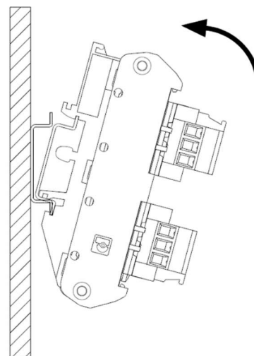
Figura 2.3 – Montagem do VBP10 em trilho DIN.
